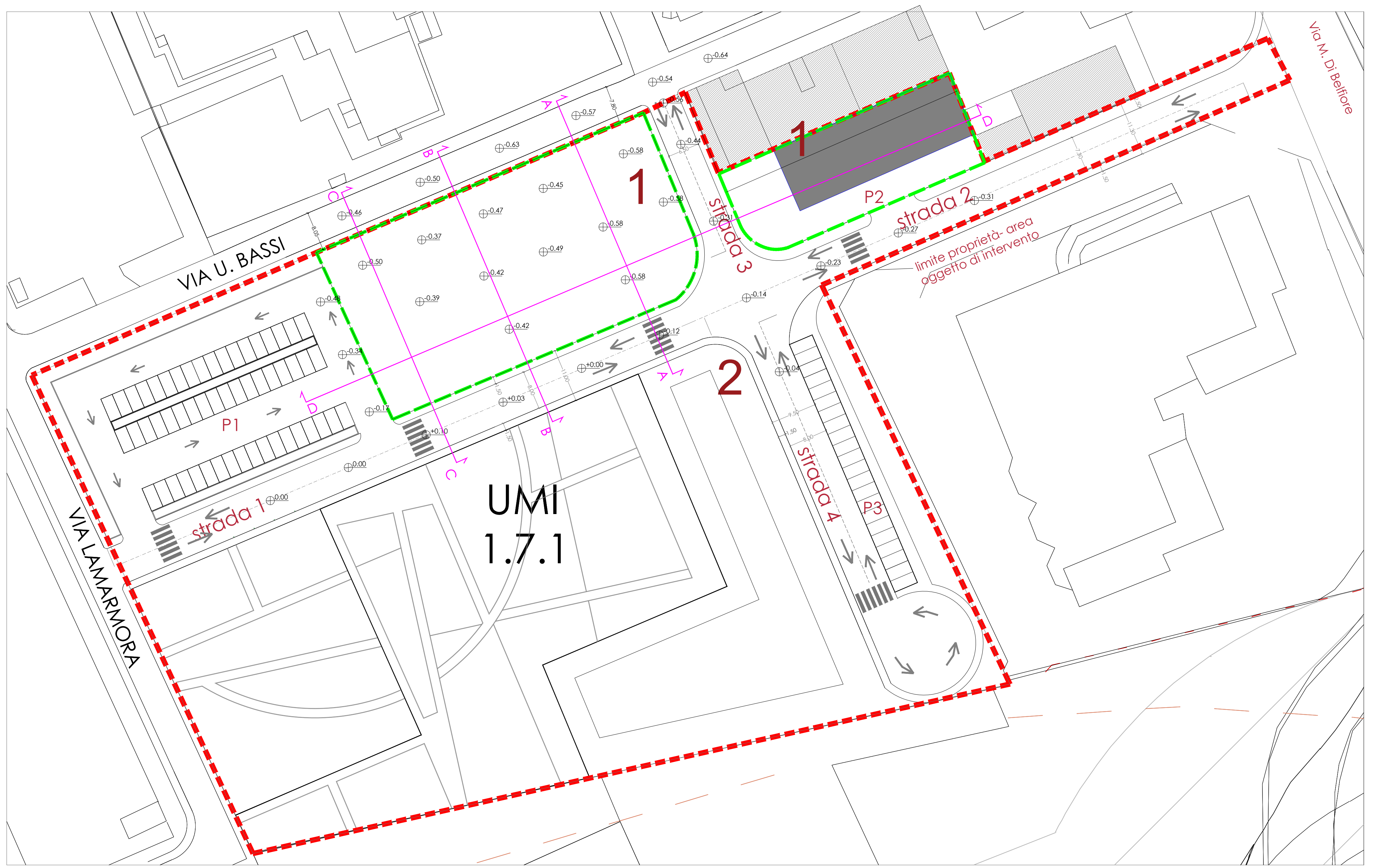
- Planimetria generale stato attuale - Scala 1:200 -
