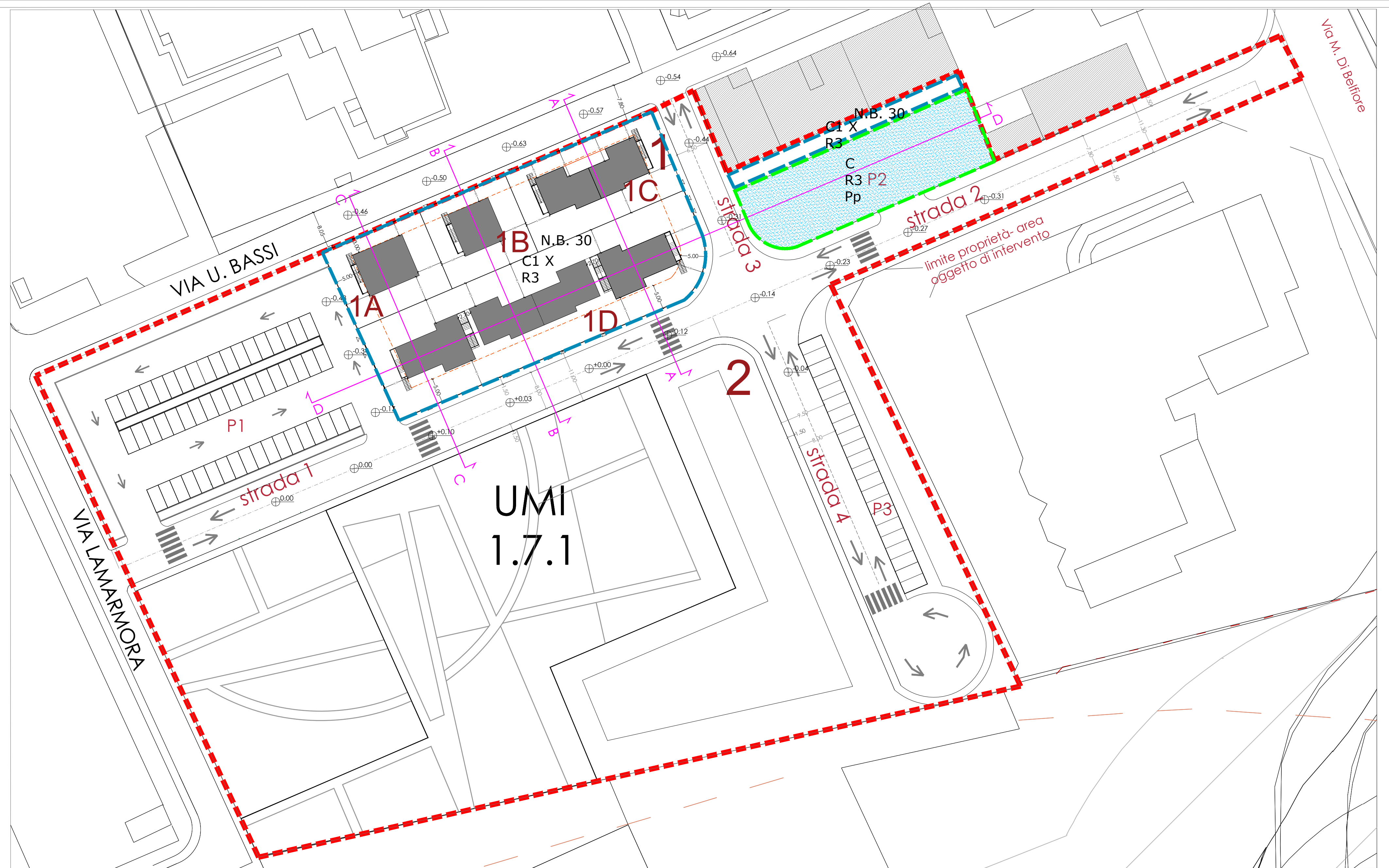
PLANIMETRIA SCALA 1:500
