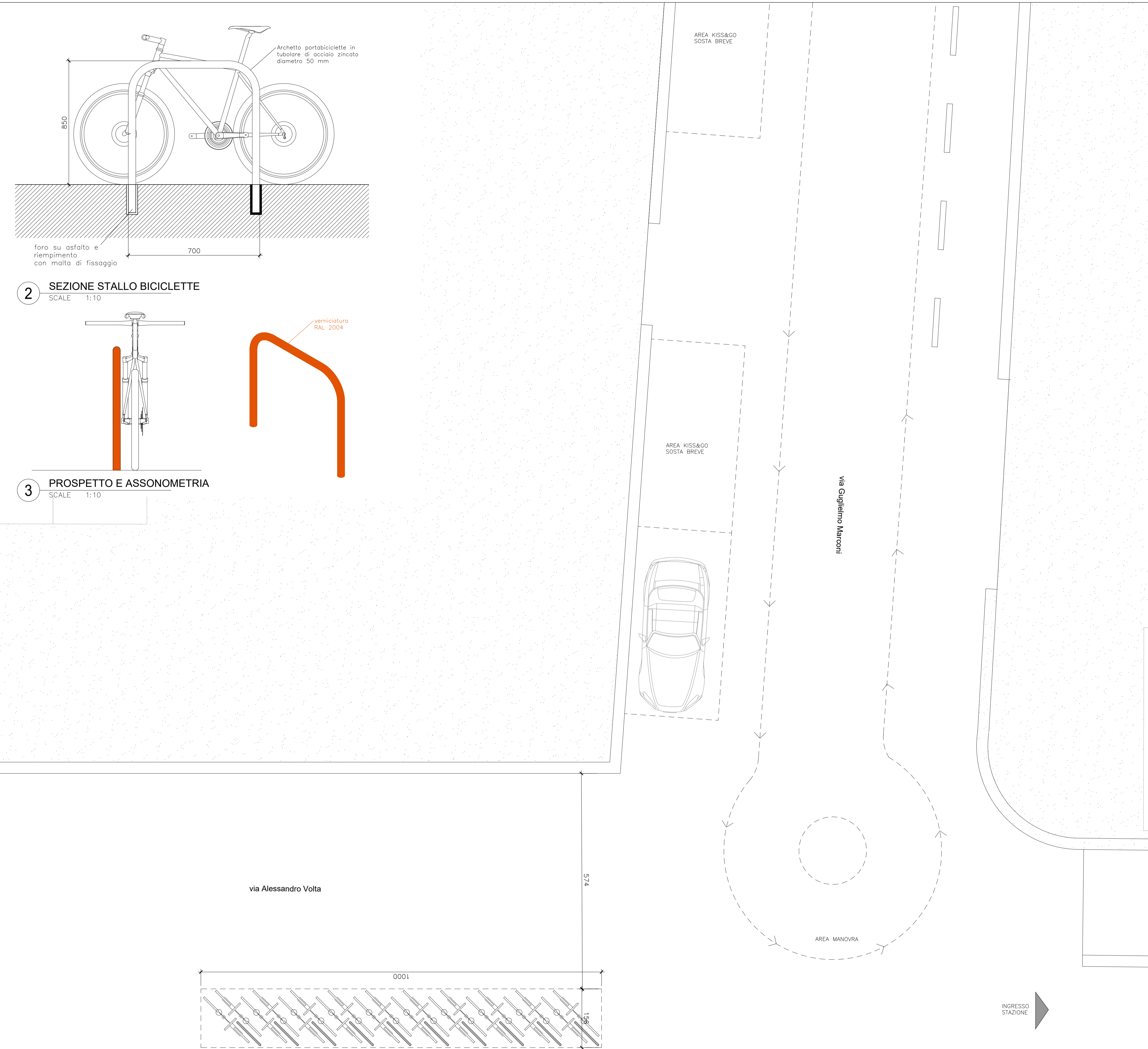
1 PLANIMETRIA STAZIONE SCALE 1:200
