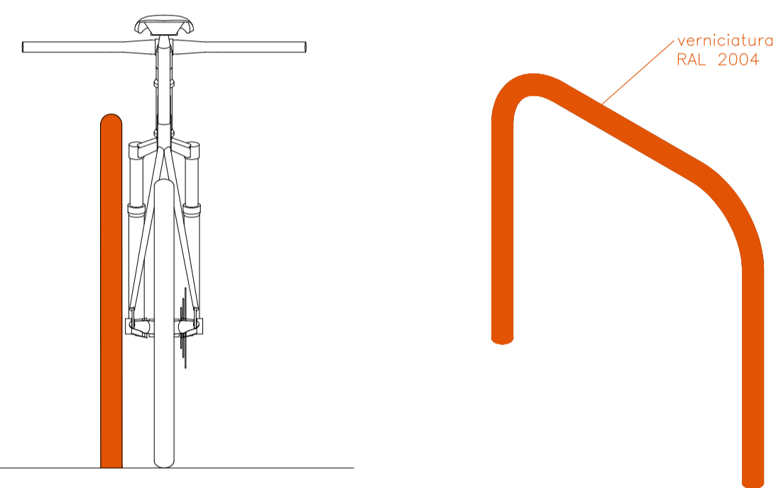
3 PROSPETTO E ASSONOMETRIA SCALE 1:10
