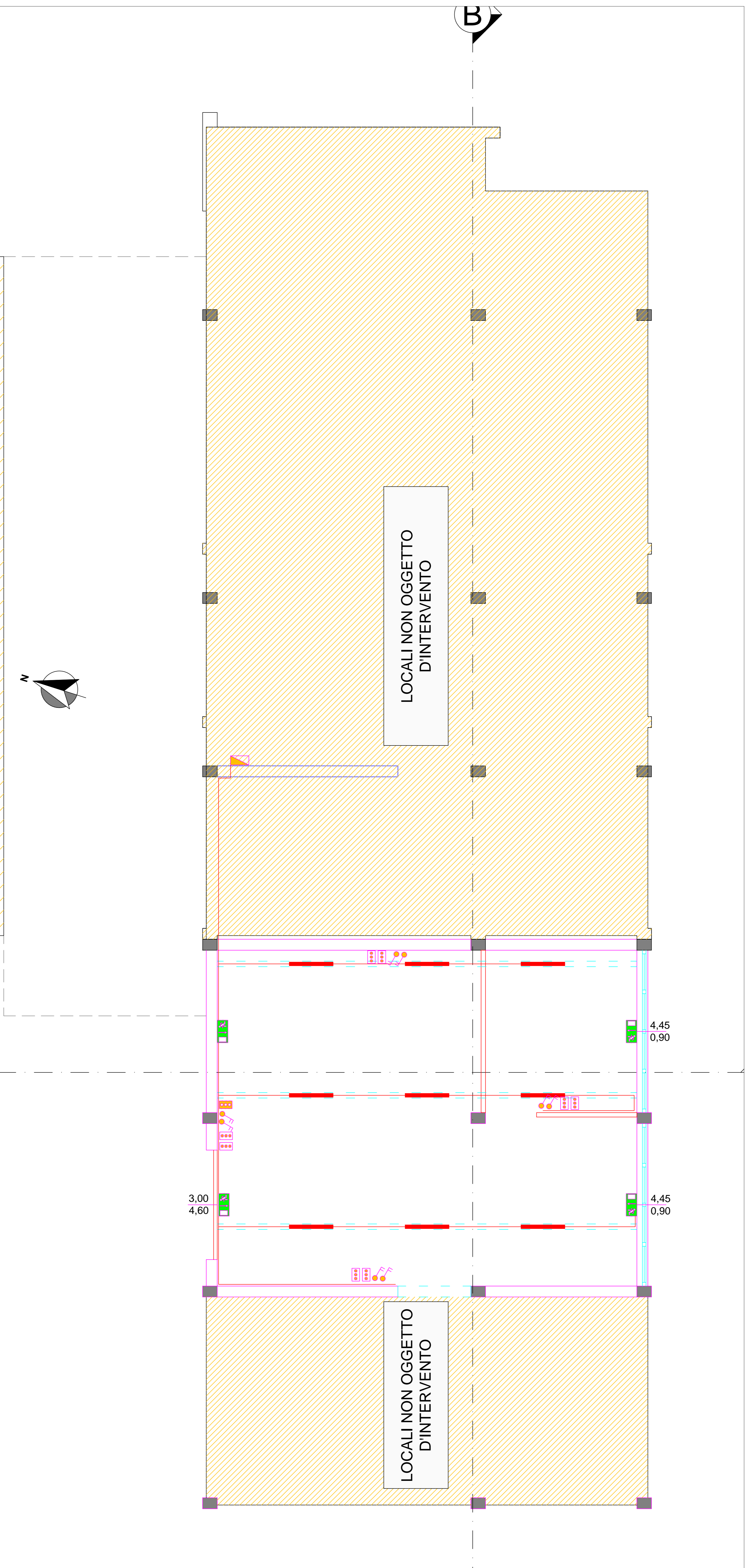
PLANIMETRIA IPOTESI DISPOSIZIONE IMPIANTO ELETTRICO scala 1:50
