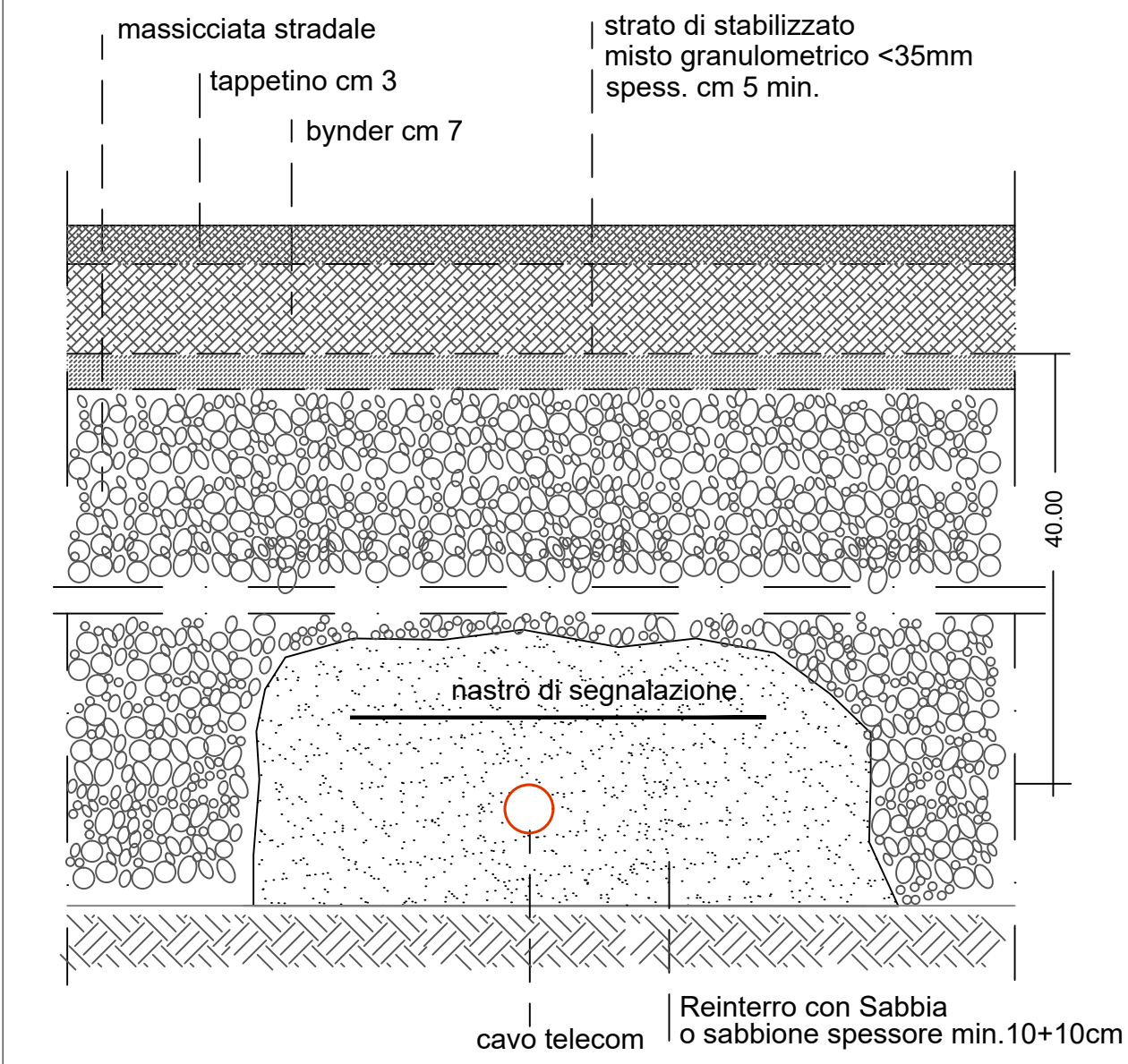
Particolare sezione tipo su marciapiede interramento canalizzazione per linea telecom
