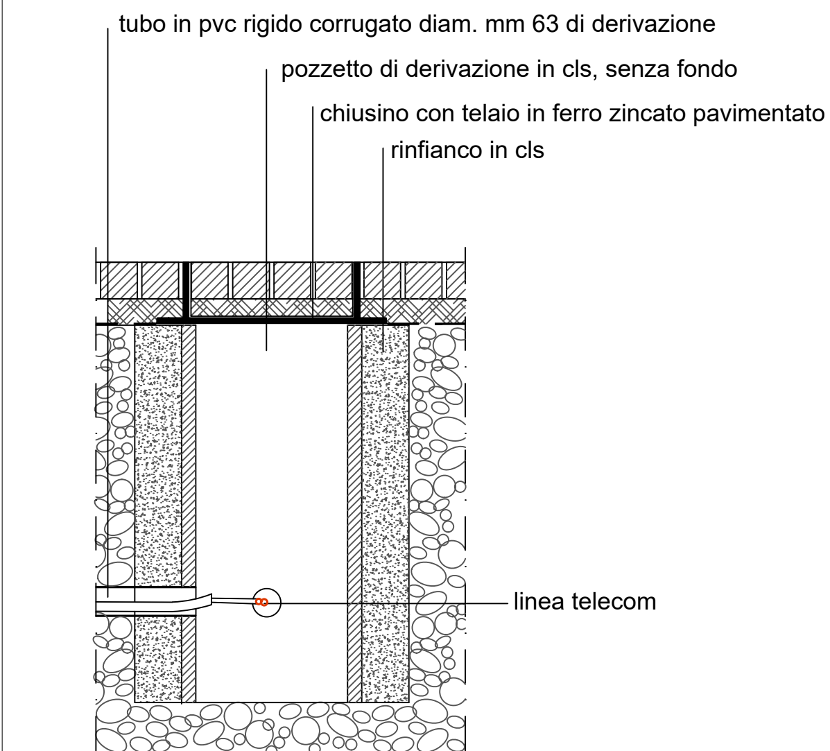
Particolare sezione tipo su piazzale pozzetto di derivazione linea telecom, in cls senza fondo
